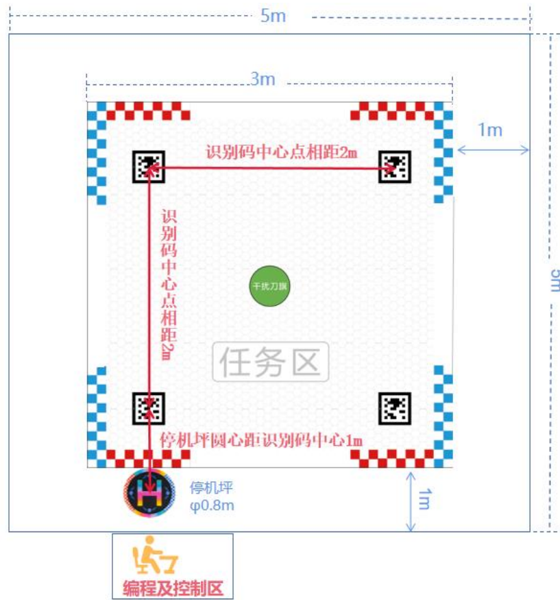
场地示意图
